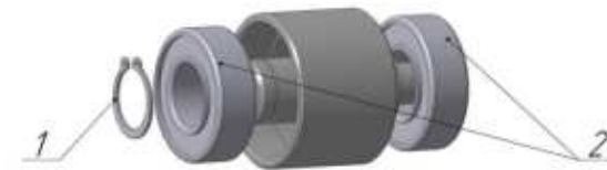
Рисунок 6. Ролик натяжной УМДУ-80/82.02.09
