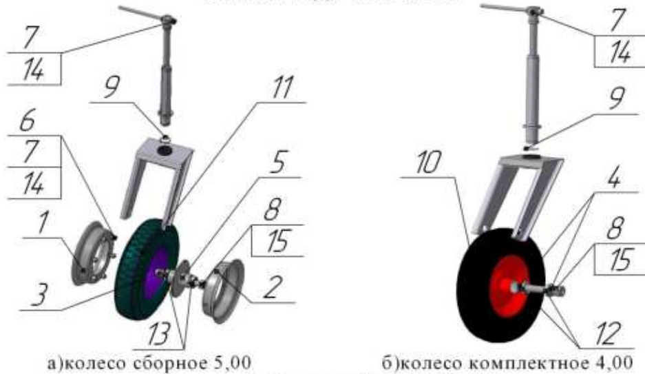
Рисунок 5. Колесо УМДУ-80/82.02.06
